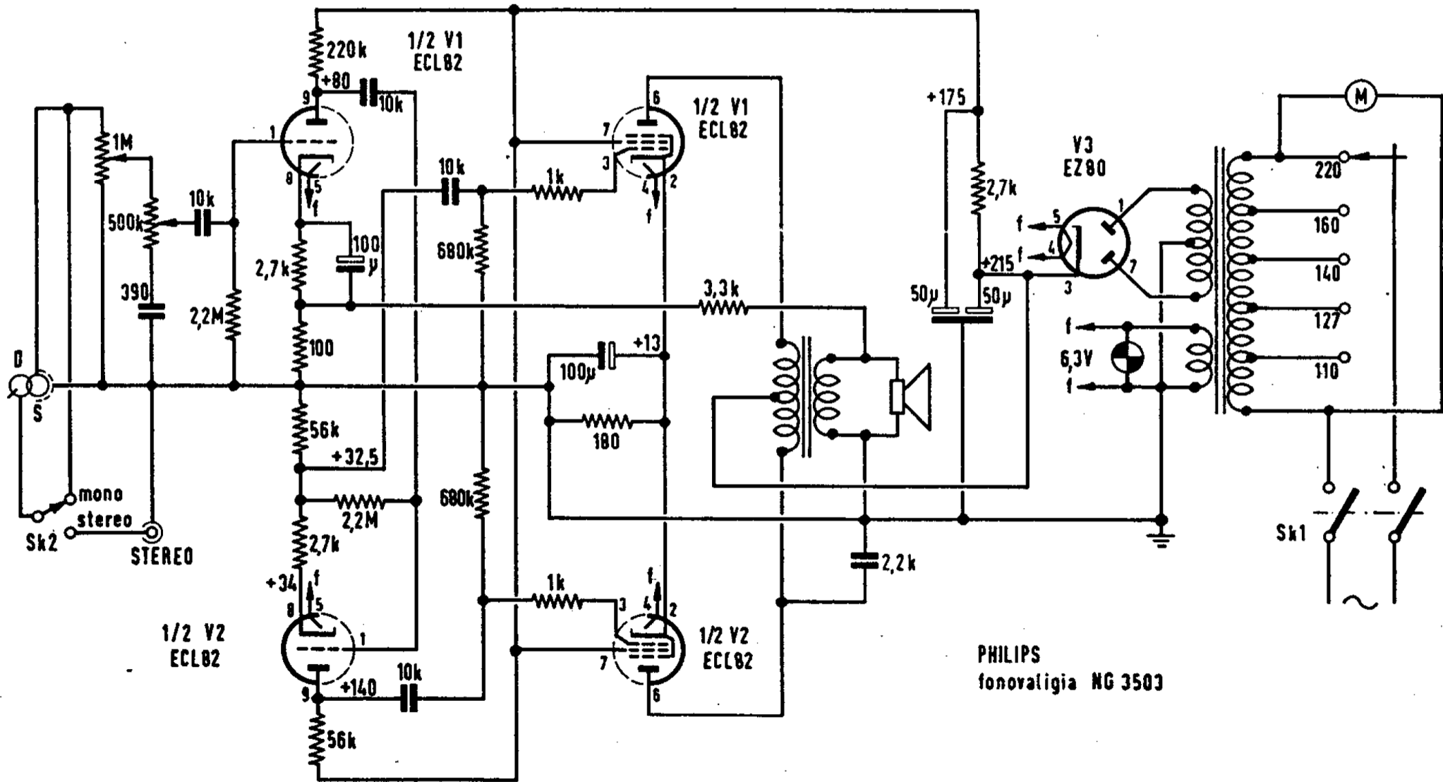
Schema elettrico della fonovaligia PHILIPS, mod. NG 3503
